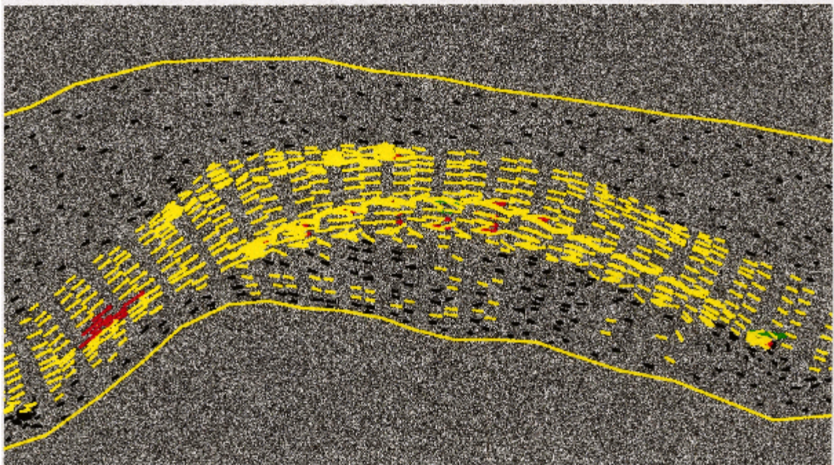
Ausbauvariante mit Buhnen
